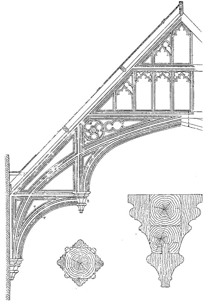
Rácsmervítéses tetőszékek.
