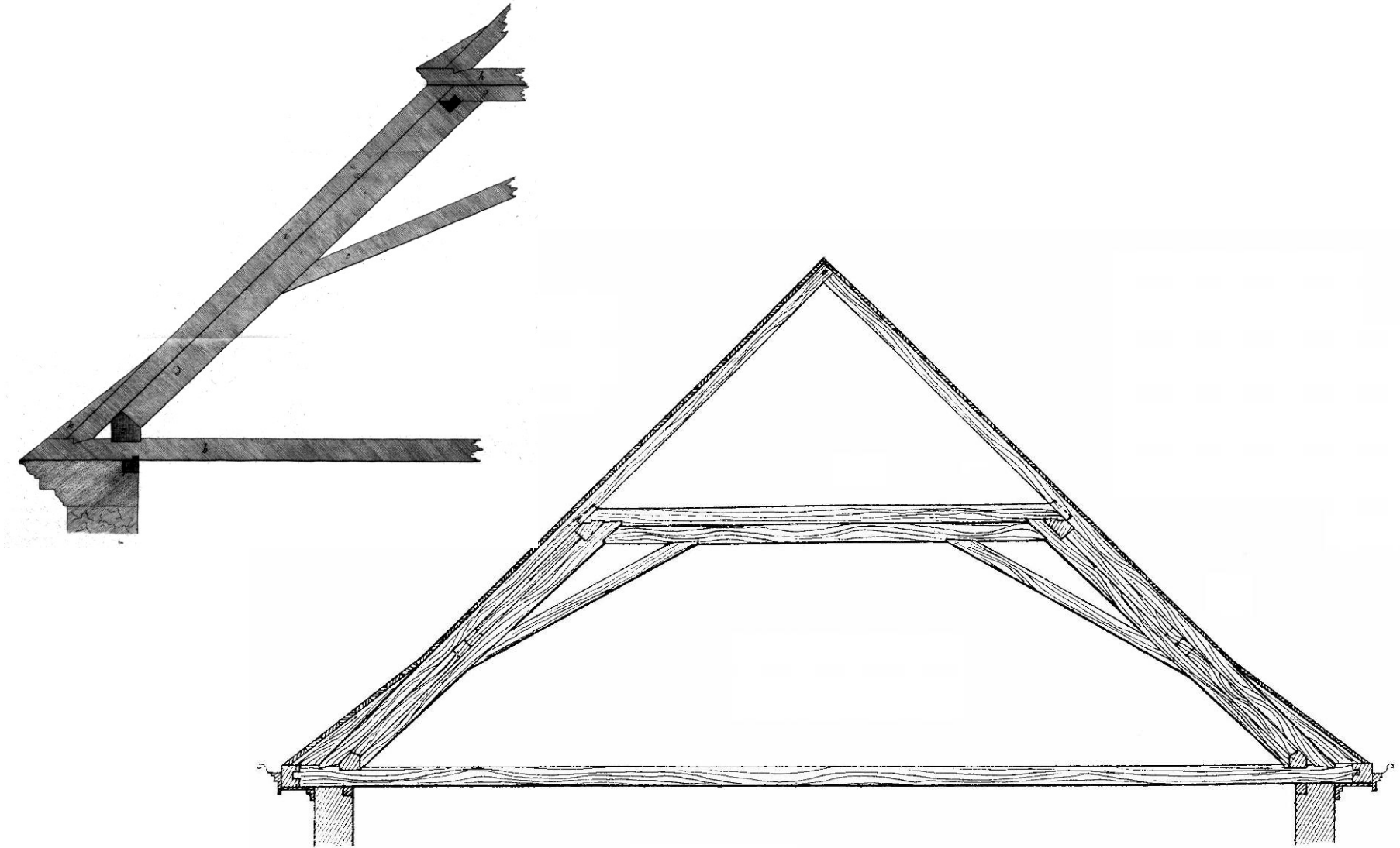
Feszítőbordás (barokk) fedélszék.
