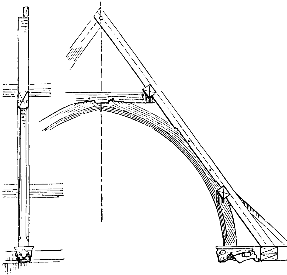
Ívmerevítő szerkezet.
