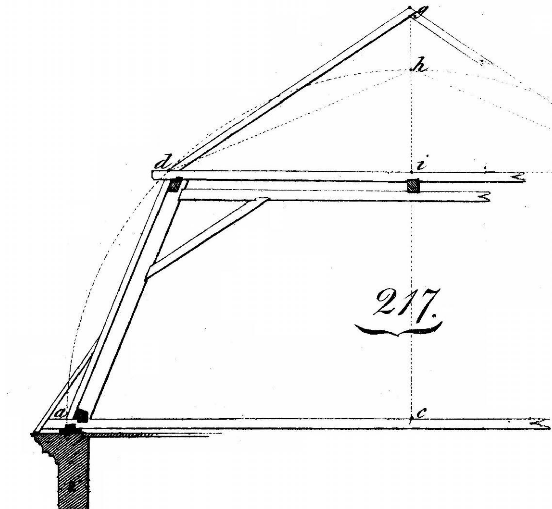
Barokk manzárdos fedés: torokgerendás és hónaljás fedélszék .
